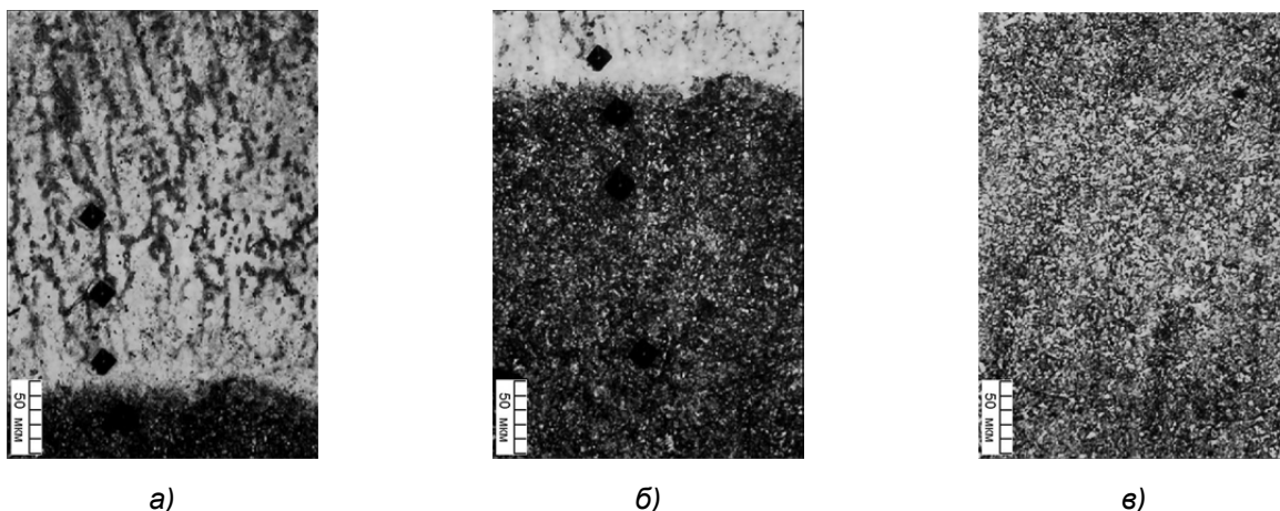
Рисунок 2. — Изменение микроструктуры после наплавки стальным электродом на подогретую до 300\,^{\circ}\text{C} основу подложки, \times 400 : а — структура наплавленного слоя (дендриты первичного твердого раствора, закаленного на мартенсит в смеси с остаточным аустенитом и частичным распадом твердого раствора по границам дендритных ветвей с выделением карбидной фазы и троостита); б — микроструктура границы сплавления и подложки, прилегающей к границе (смесь из мартенсита игольчатой морфологии, остаточного аустенита и троостита); в — микроструктура подложки по мере углубления от сплавления (смесь из мартенсита, остаточного аустенита, троостита и цепочек цементита по границам бывших аустенитных зёрен)
