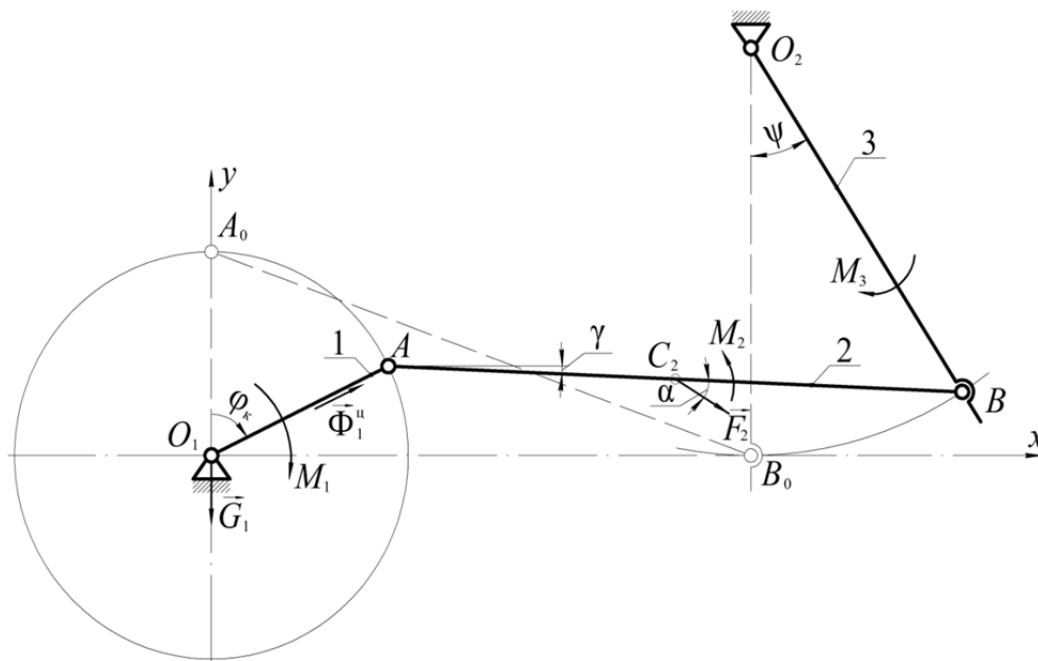
Рисунок 1. — Схема механизма с действующими на него внешними силами
