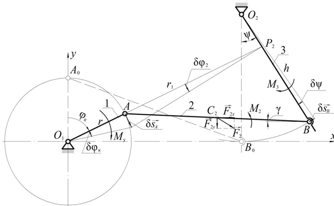
Рисунок 4. — Разлікова схема для визначення M_y
