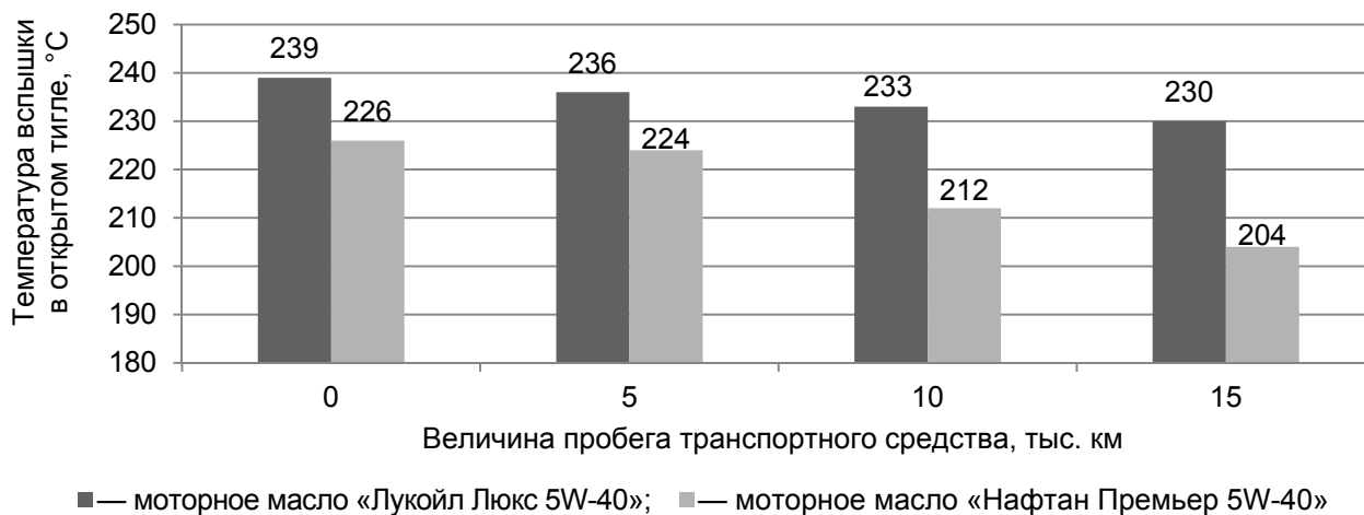
Рисунок 2. — Изменение температуры вспышки в открытом тигле синтетических моторных масел при увеличении величины пробега транспортного средства
