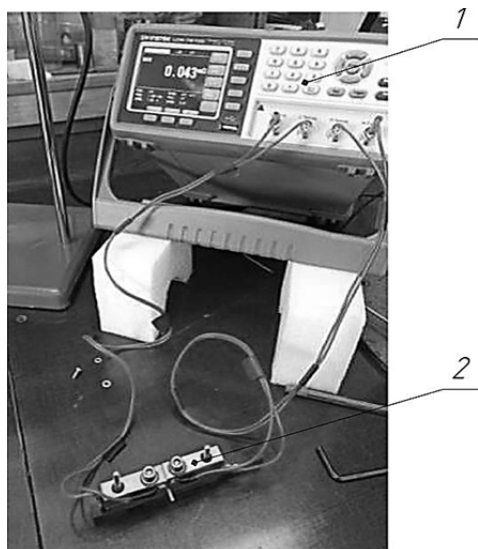
Рисунок 2. — Стенд для измерения удельного сопротивления
