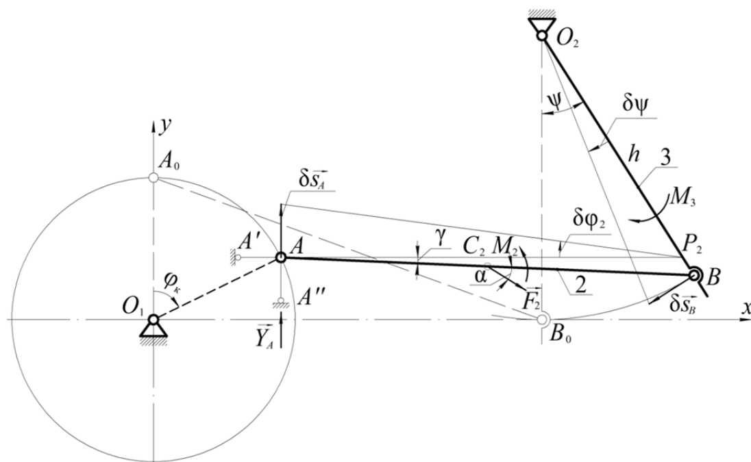
Рисунок 6. — Разрізова схема для визначення компонента Y_A
