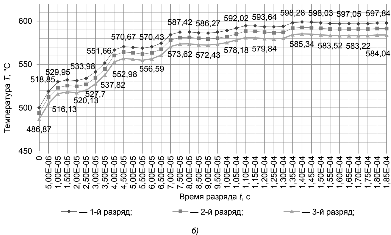
Рисунок 1. — Зависимость максимальной температуры нагрева от времени разряда: а — при полной загрузке сверла; б — при половинной загрузке сверла
