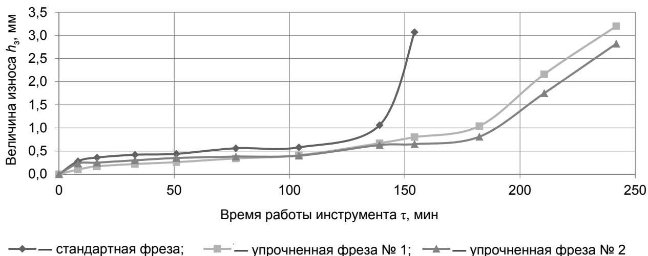
Рисунок 7. — Зависимости величины износа по задней поверхности фрез, обработанных аэродинамическим звуковым методом
