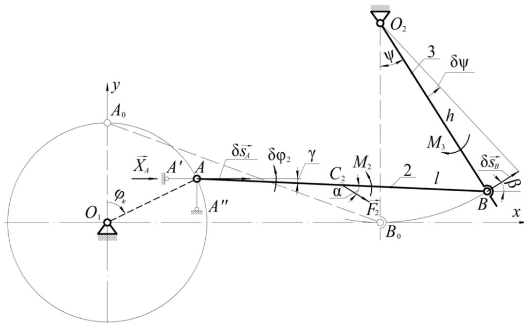
Рисунок 5. — Разрізова схема для визначення компонента X_A
