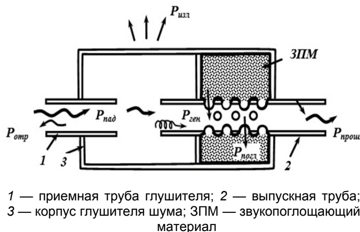
Рисунок 1. — Распределение потоков звуковой энергии в глушителе
