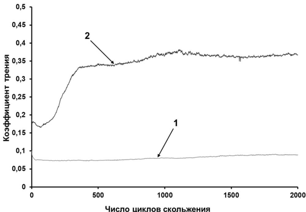
1 — твердый сплав ВК6 после ТГХО в оптимальном режиме и составе на базе ZnO + MoO_3 ; 2 — исходный твердый сплав ВК6 (без обработки)
