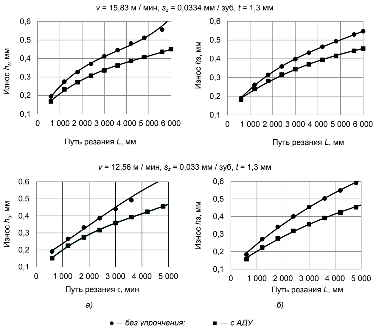
Рисунок 13. — Зависимости износа по задней поверхности h_3 , полученные экспериментально и рассчитанные по формулам, для концевых фрез Р6М5, упрочненных АДУ и неупрочненных, от пути резания при фрезеровании стали 45: а — зависимости экспериментальные; б — зависимости, построенные по формулам
