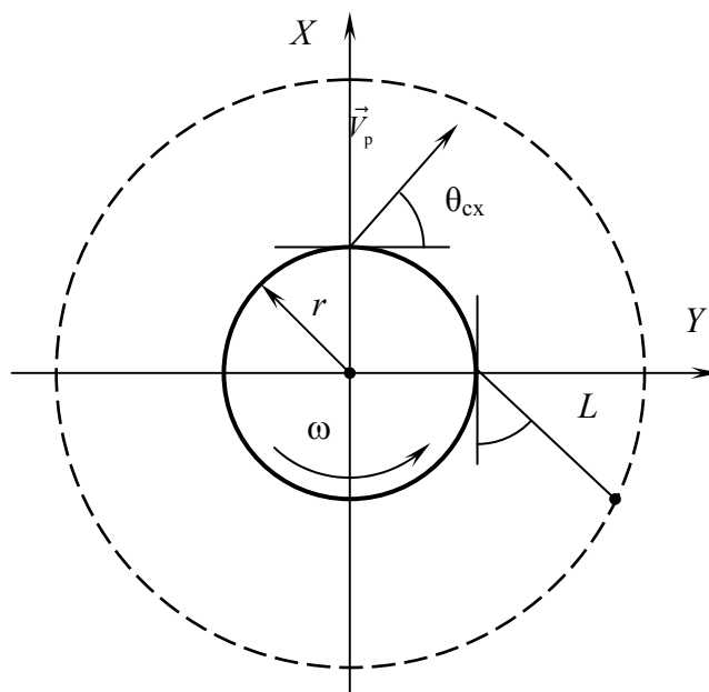
Рисунок 5. — Геометрическое место распределения частиц по поверхности поля при неподвижной машине с учетом дальности полета частиц L , радиуса диска r , угла схода \theta_{cx} и начальной скорости V_p
