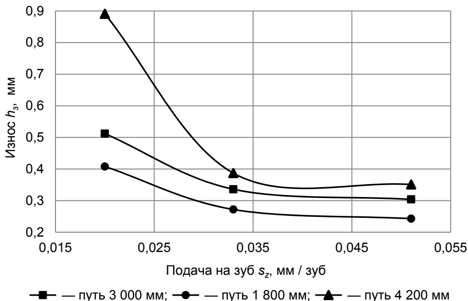
Рисунок 9. — Зависимости износа h_3 зуба фрезы диаметром 8 мм из Р6М5 с АДУ при фрезеровании стали 45 от поддачи s_z при путях резания L : 1 800; 3 000; 4 200 мм ( v = 15,83 м / мин, t = 1,3 мм)
