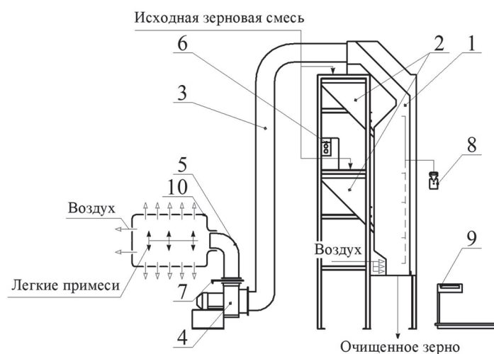
1 — лабораторный макет пневматического канала окончательной асирации МУЗ-16; 2 — бункера для исходной зерновой смеси; 3, 5 — воздуховод; 4 — вентилятор; 6 — магнитный пускатель двигателя вентилятора; 7 — заслонка; 8 — термоанометр; 9 — весы; 10 — фильтровальная перегородка
