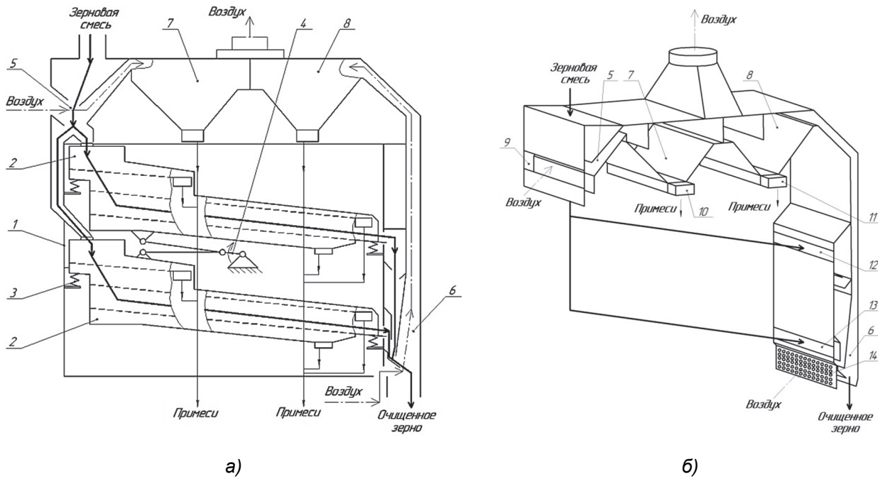
1 — корпус; 2 — ситовые кузова; 3 — виброопоры; 4 — приводной эксцентриковый механизм; 5 — пневматический канал предварительной асирации; 6 — пневматический канал окончательной асирации; 7, 8 — осадочные камеры; 9, 14 — входы воздуха в пневматические каналы; 10, 11 — выходы примесей из осадочных камер; 12, 13 — входы зерновой смеси в пневматический канал окончательной асирации
