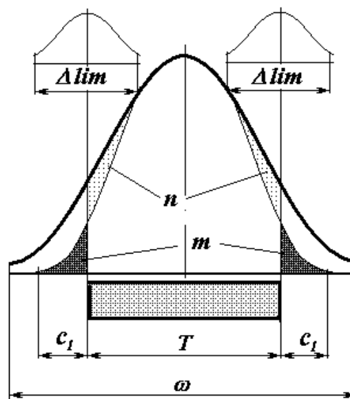
Рисунок 1. — Схема контроля
