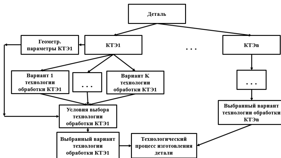
Рисунок 6. — Схема формирования технологического процесса изготовления детали методом структурного синтеза
